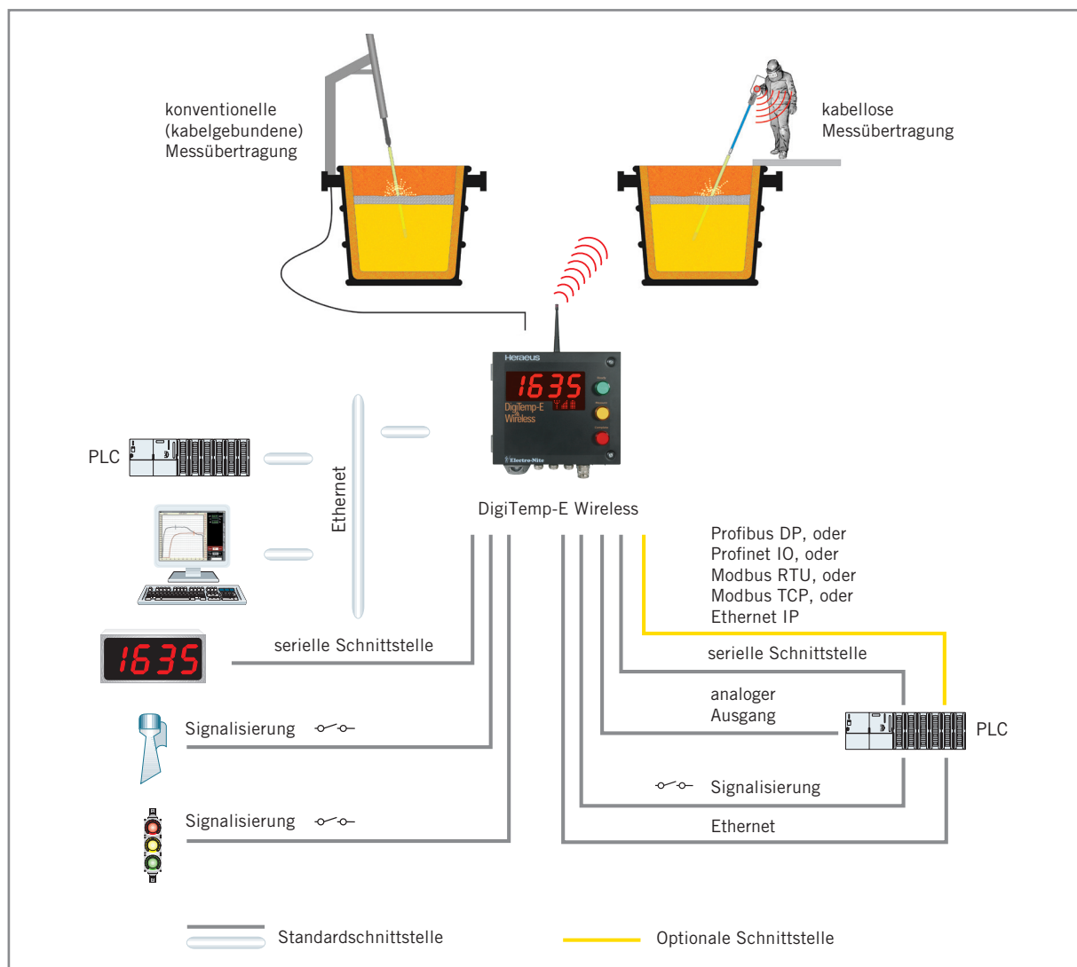
DigiTemp-E Wireless mit Standardschnittstellen und optionalen Schnittstellen
